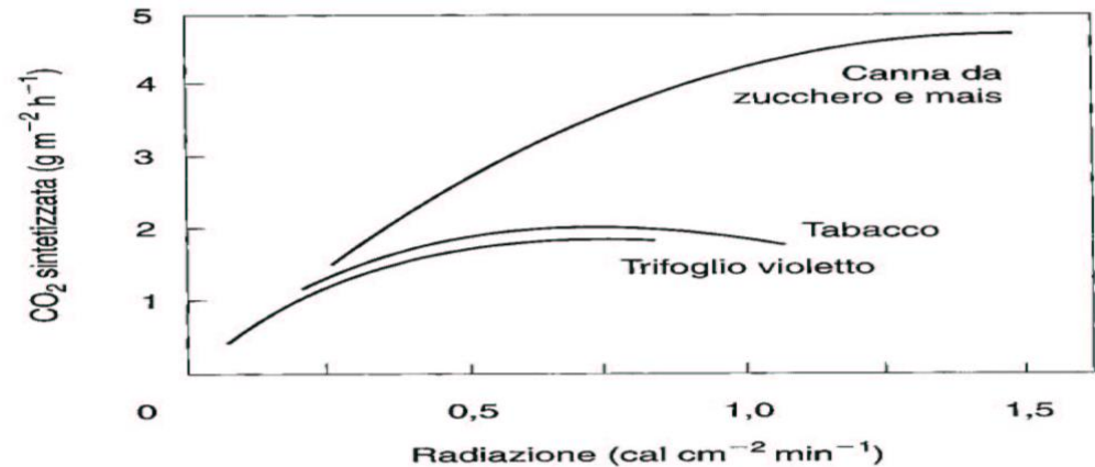
Fig. 2.4 Assorbimento della CO 2 in funzione dell'intensità di radiazione.
